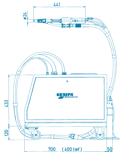
GAV-7000 con pistola de remachado Robotica
